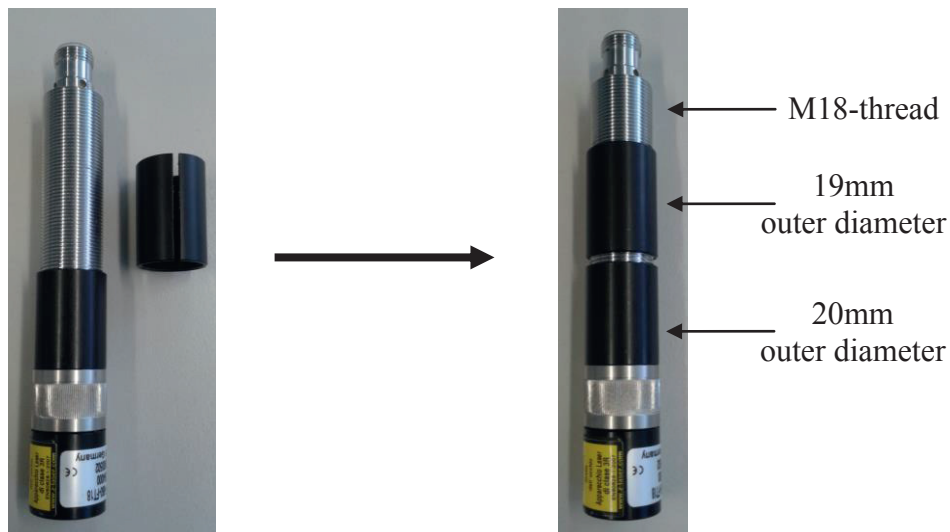
ZM18S3-laser + AP-M18-19
